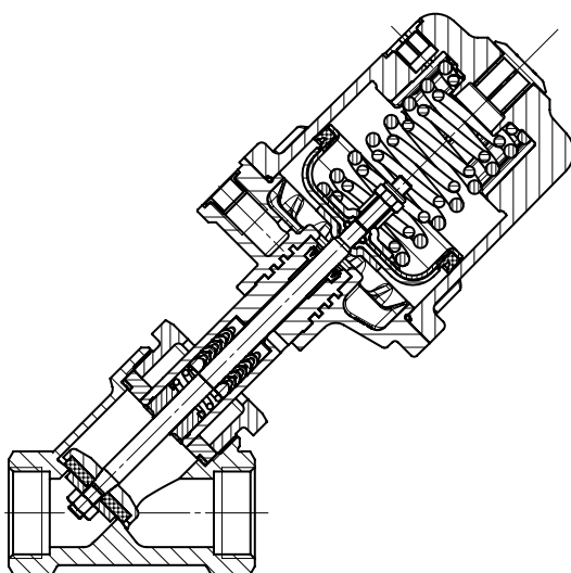
Výkres řezu
