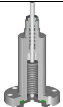
BONNET with BELLOWS BONNET con SOFFIETTO
