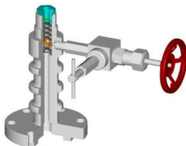
FINNED BONNET BONNET ALETTATO
