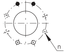
DN350 - DN400
