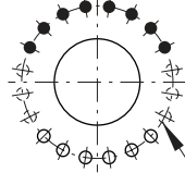
DN500
